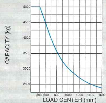
FD45T9·C9 (5000kg)
