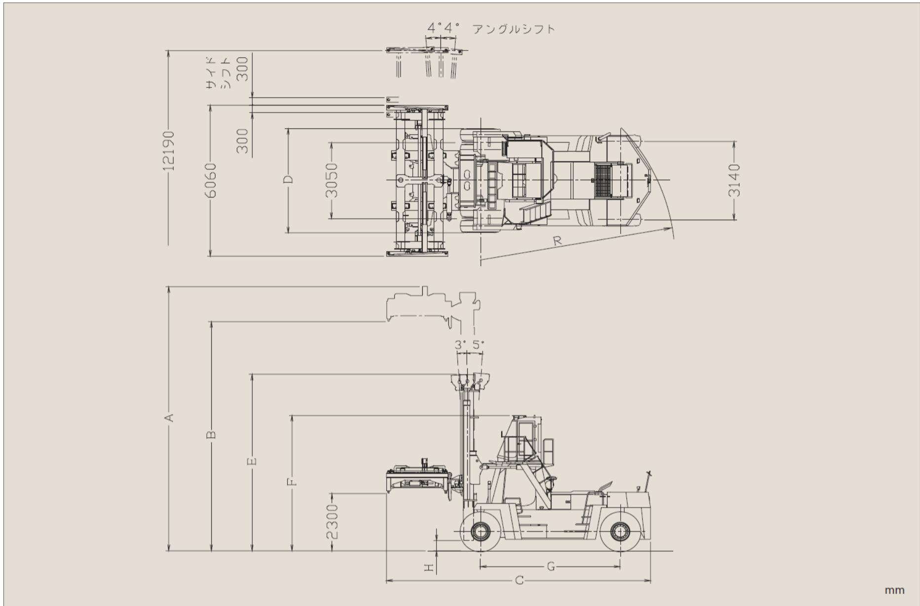
外形寸法図
